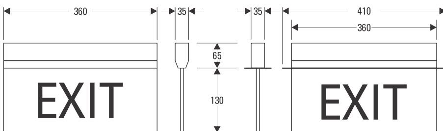
Surface type dimensions (mm) Kích thước loại gắn nổi
