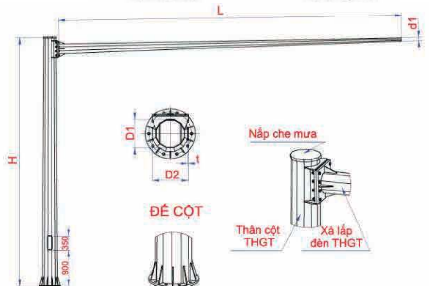
Mặt cắt thân cột
