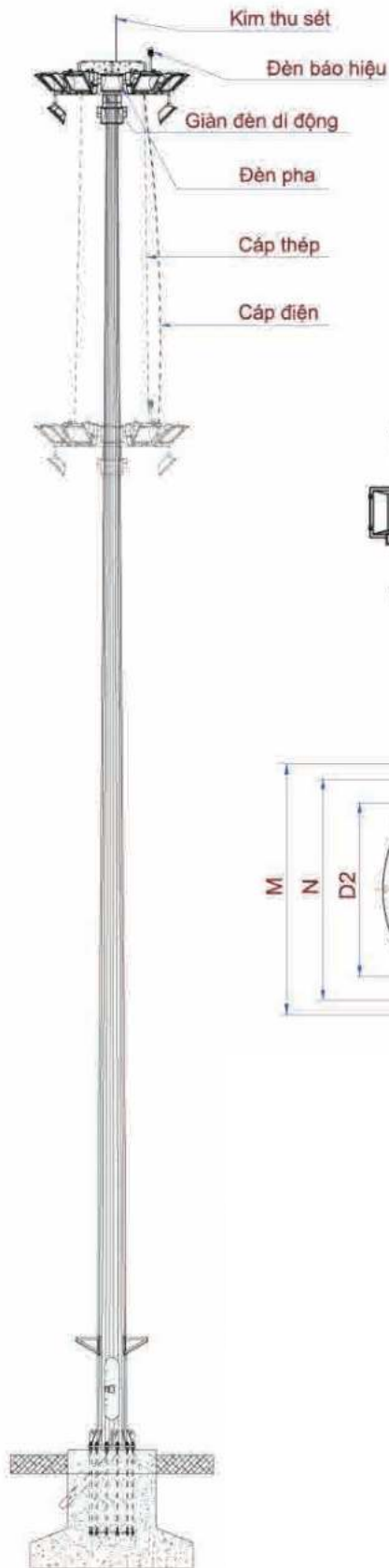
Bố trí đèn pha
